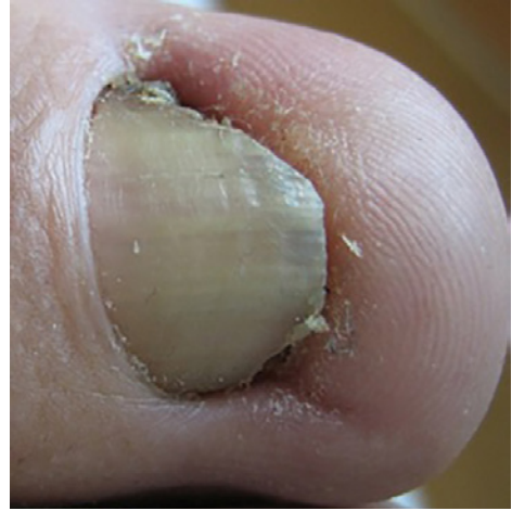
Abb. 2.41 Falscher Nagelschnitt
